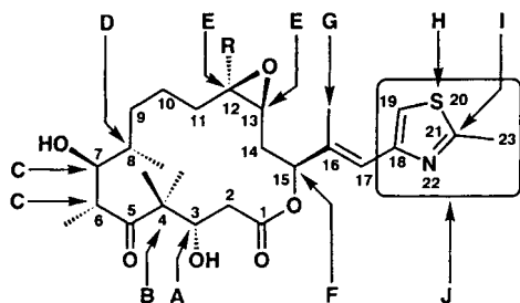
Schema 2. Struktur-Wirkungs-Beziehungen (Tubulin-Bindungsassay) der Epothilone: A) (3 S )-Konfiguration ist wichtig; B) 4,4-Ethanogruppe wird nicht toleriert; C) (6 R ,7 S )-Konfiguration ist entscheidend; D) (8 S )-Konfiguration ist wichtig, 8,8-Dimethylfunktionalität wird nicht toleriert; E) Epoxid ist nicht essentiell für Tubulin-Polymerisations-Aktivität, aber eventuell wichtig für Cytotoxizität; Epoxid-Konfiguration ist möglicherweise wichtig; Rest R ist wichtig; beide Olefin-Geometrien werden toleriert; F) (15 S )-Konfiguration ist wichtig; G) sterisch anspruchsvollere Gruppe verringert Aktivität; H) Sauerstoffs substituent wird toleriert; I) Substituent ist wichtig; J) Heterocyclus ist wichtig.
